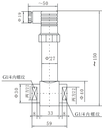
图 1 接插件型
