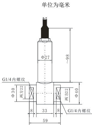
图 2 电缆型
