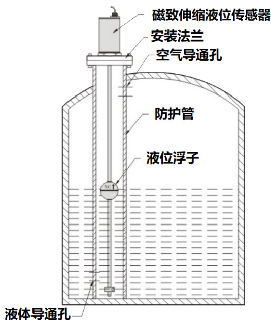
图一 防护管安装方法示意图
