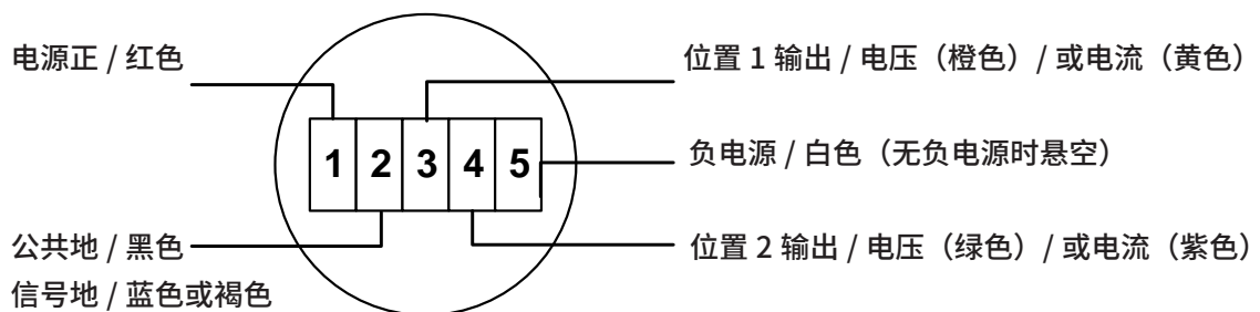
双位置输出接线端子接线图
