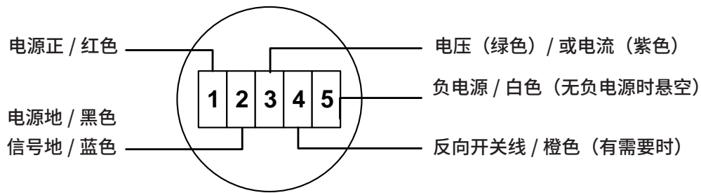
单位置输出接线端子接线图
