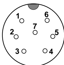
公插头 (磁尺连接端)
