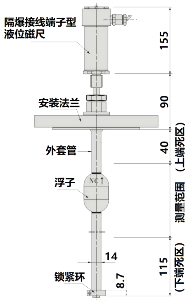
图三 带压容器专用型
