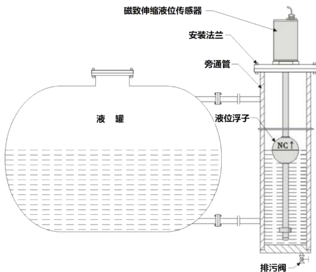
图二 旁通管安装方法示意图
