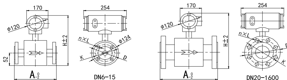
图 2 一体式外形尺寸
