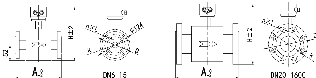
图 3 分体式外形尺寸
