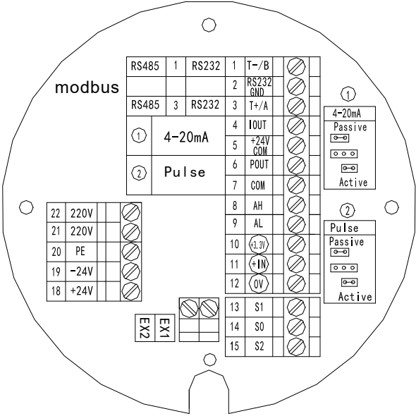
图 5 一体式接线图
