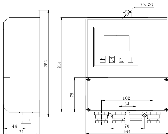
图 4 分体式转换器尺寸
