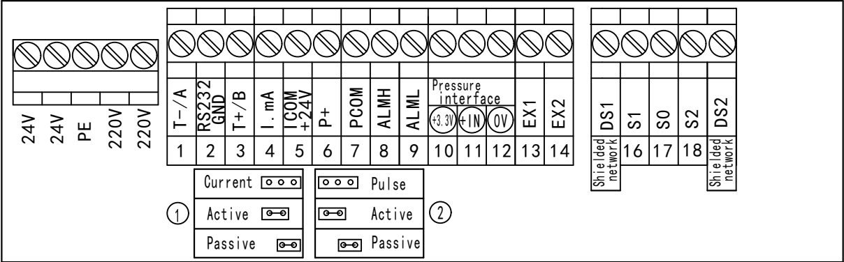
图 6 分体式接线图
