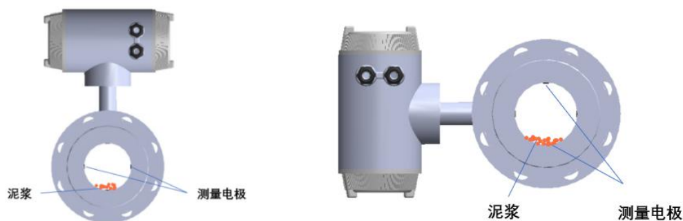
图 13 流量计安装方向
