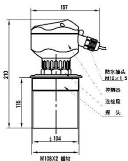
M108×2 螺纹传感器
