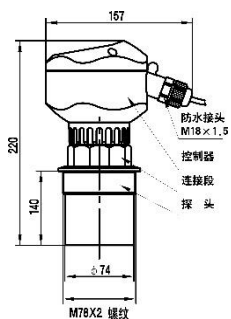
M78×2 螺纹传感器
