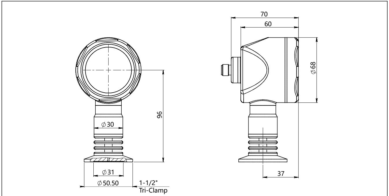
高温型带显示 (C) /不带显示 (A) 垂直安装 (F1) 整机尺寸图 (单位: mm)
