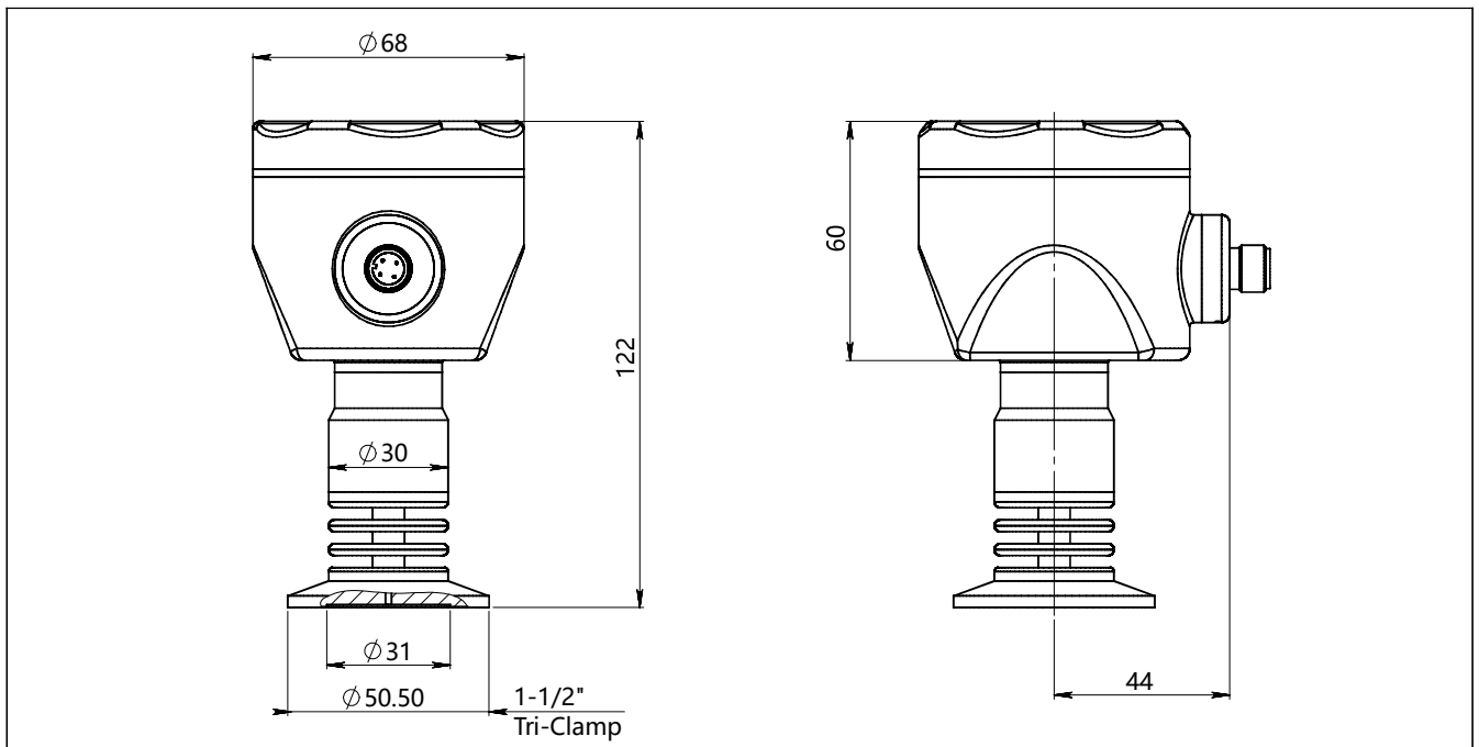
高温型带显示 (C) /不带显示 (A) 水平安装 (F2) 整机尺寸图 (单位: mm)
